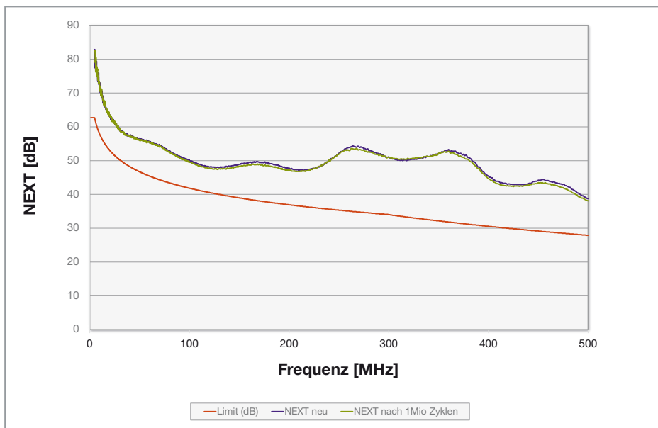
Signalübertragung neu und nach 1 Mio. Zyklen am Beispiel NEXT
