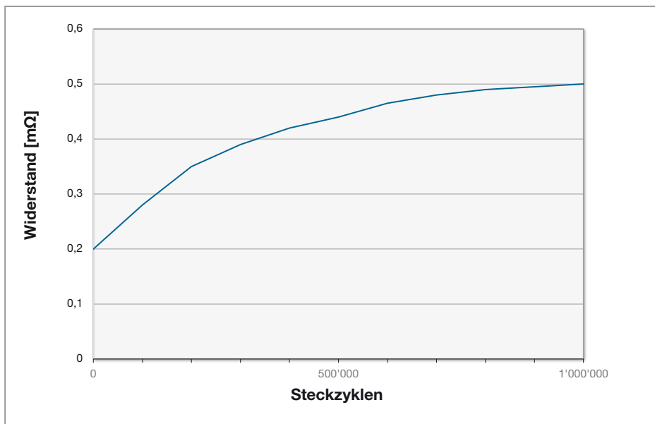
Widerstandsänderung bei Zyklen
