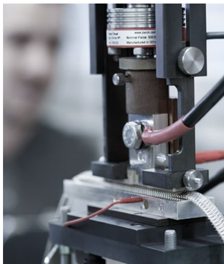
Essais des matériaux de MULTILAM : résistance à la pression
